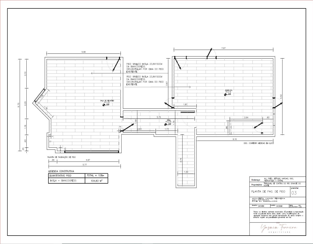
Figura 1: Planta de paginação de piso, conforme projeto aprovado.
