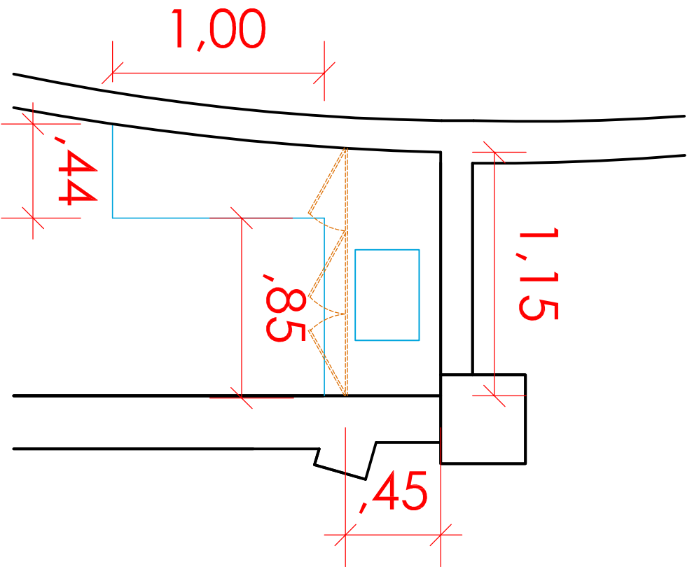
PLANTA BAIXA ARMÁRIOS COPA PLENÁRIO 01 armário superior + 01 armário em "L"
