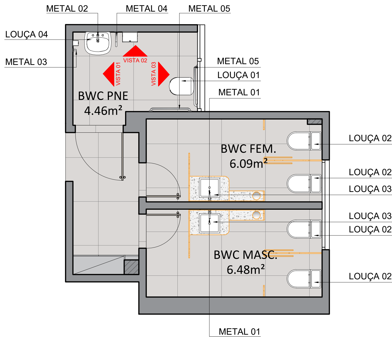
PLANTA DE LAYOUT - LOUÇAS E METAIS ESCALA.....1/40
