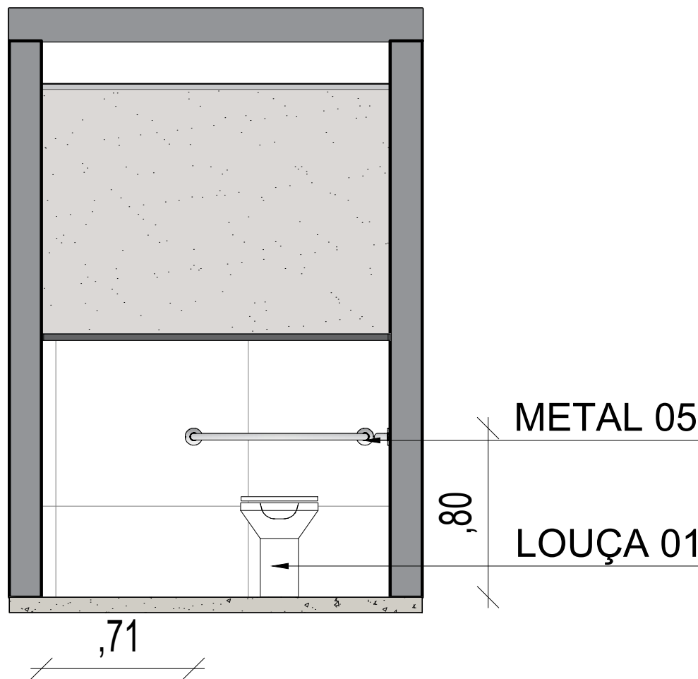
VISTA 03 ESCALA 1/25
