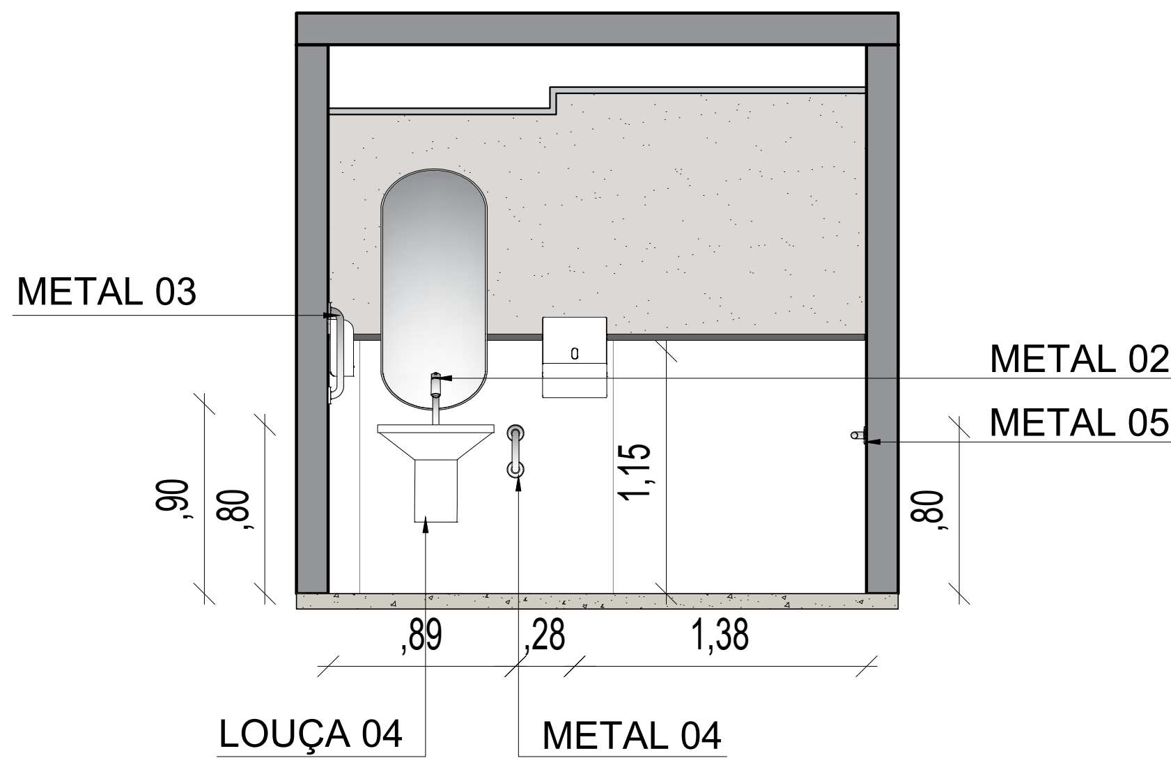
VISTA 02 ESCALA 1/25
