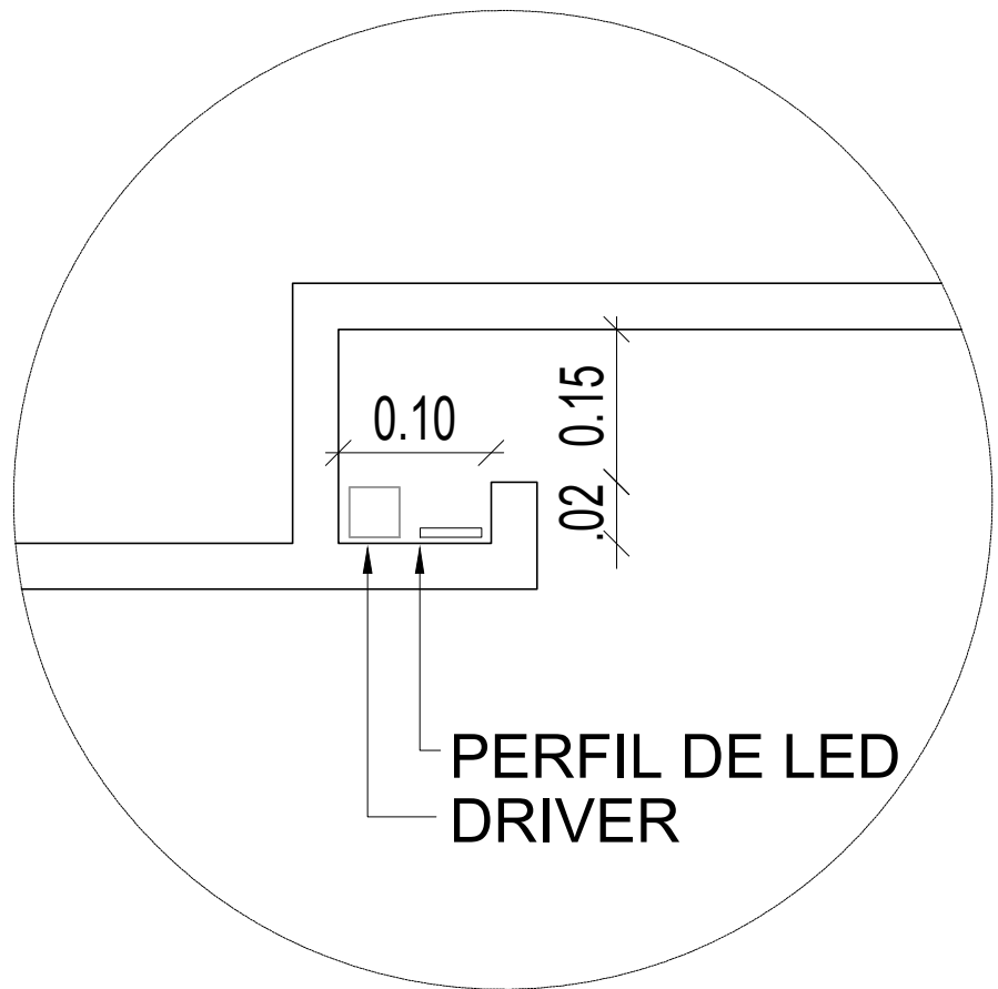
DETALHE 02 ESCALA - 1/25
