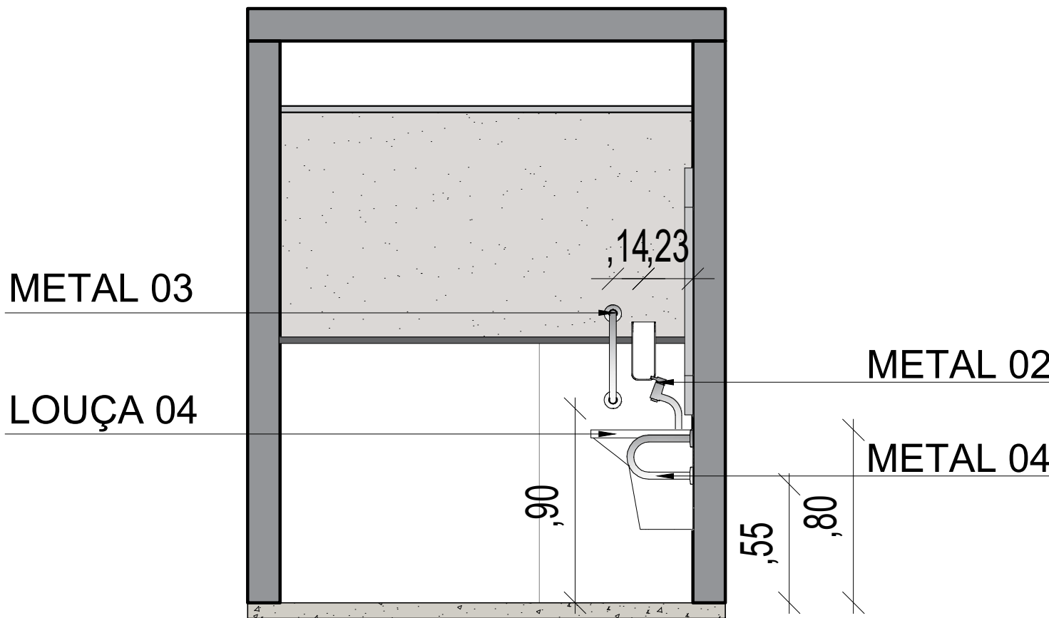
VISTA 01 ESCALA 1/25
